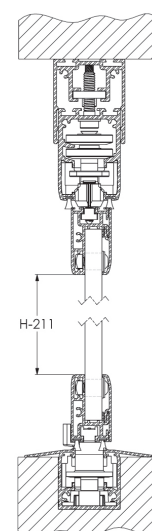
Superior con expansor Inferior embutido
