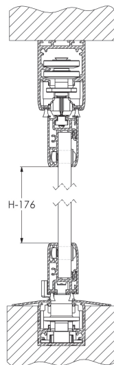
Superior sin expansor Inferior embutido
